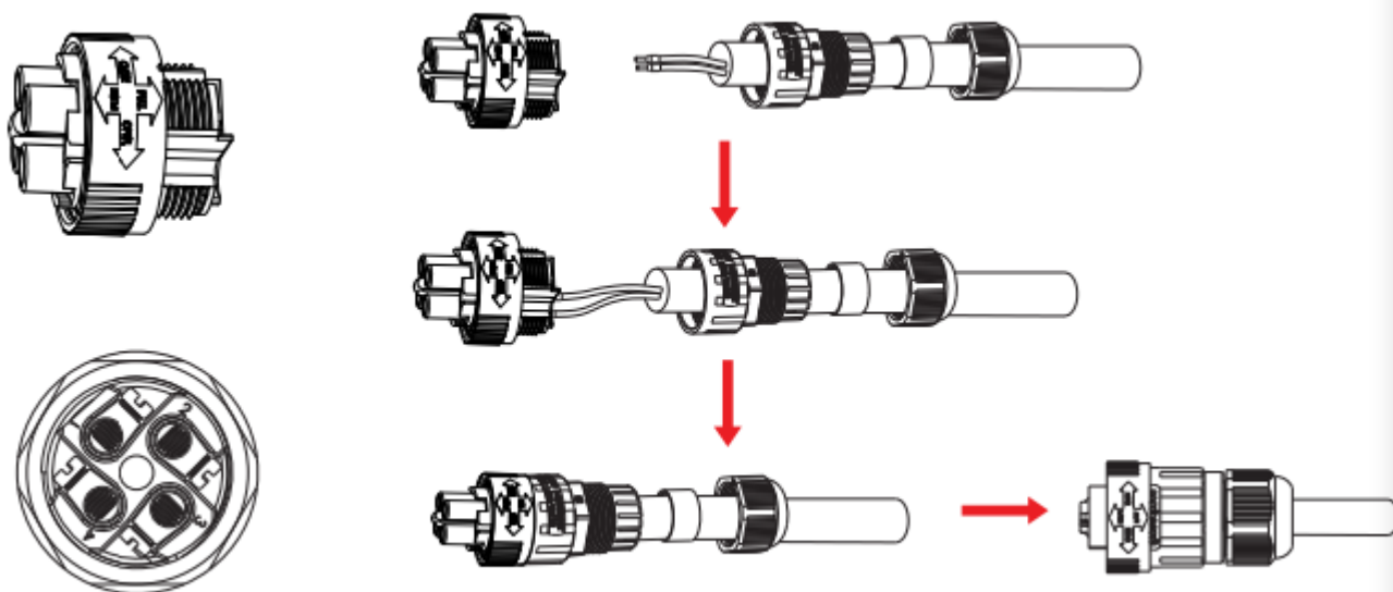
▲ Рисунок 4.23 Коннектор СТ
