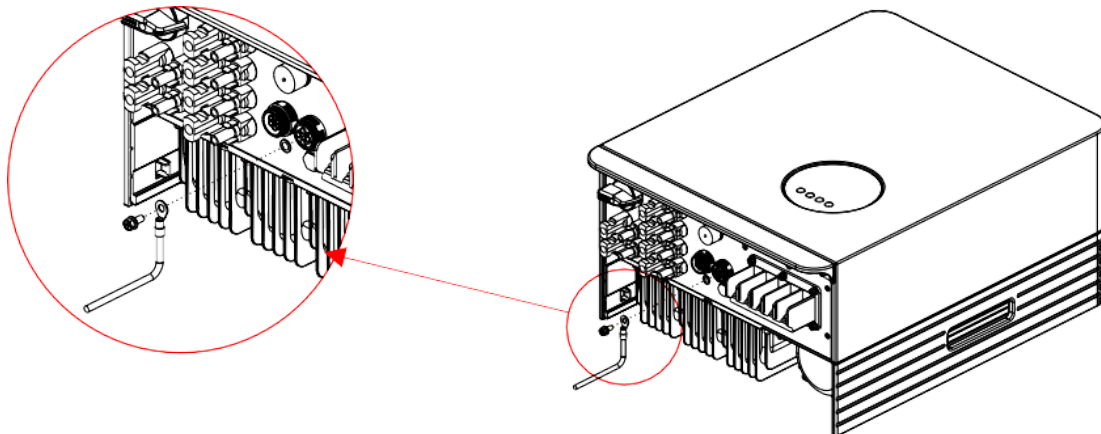
▲ Рисунок 4.19 Установка внешнего заземления
