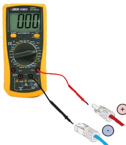
▲ Рисунок 4.6 Разъем PV+
