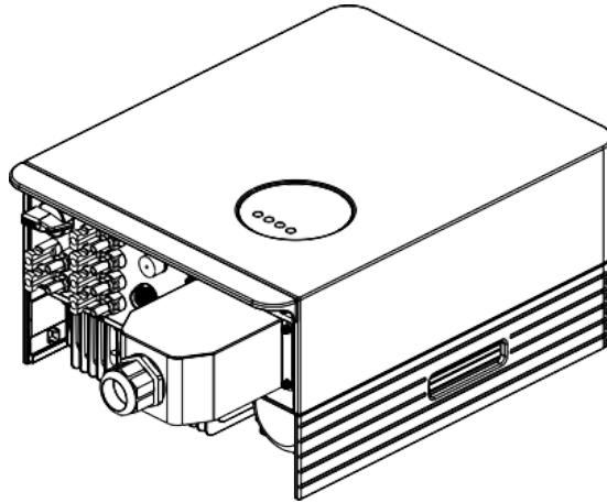
▲ Рисунок 4.18 Подключение разъема переменного тока к инвертору
